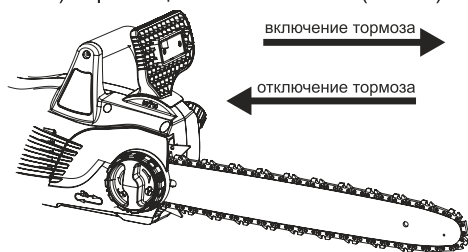
Рис. 6 Положение ручки тормоза
