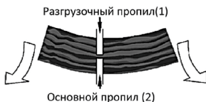
Рис. 11 Распиливание дерева, когда его нижняя часть находится под напряжением
